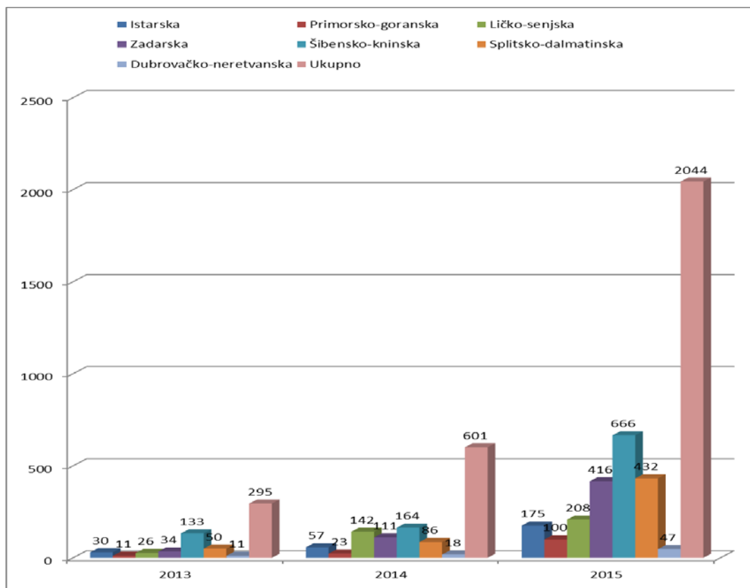
Grafikon 1. Broj požara raslinja u 2013.2014. i 2015. godini.
