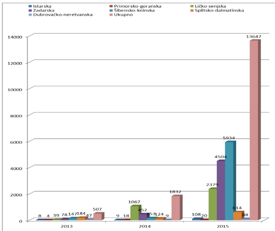
Grafikon 2. Opožarena površina u hektarima (ha) u 2013.2014. i 2015. godini.
