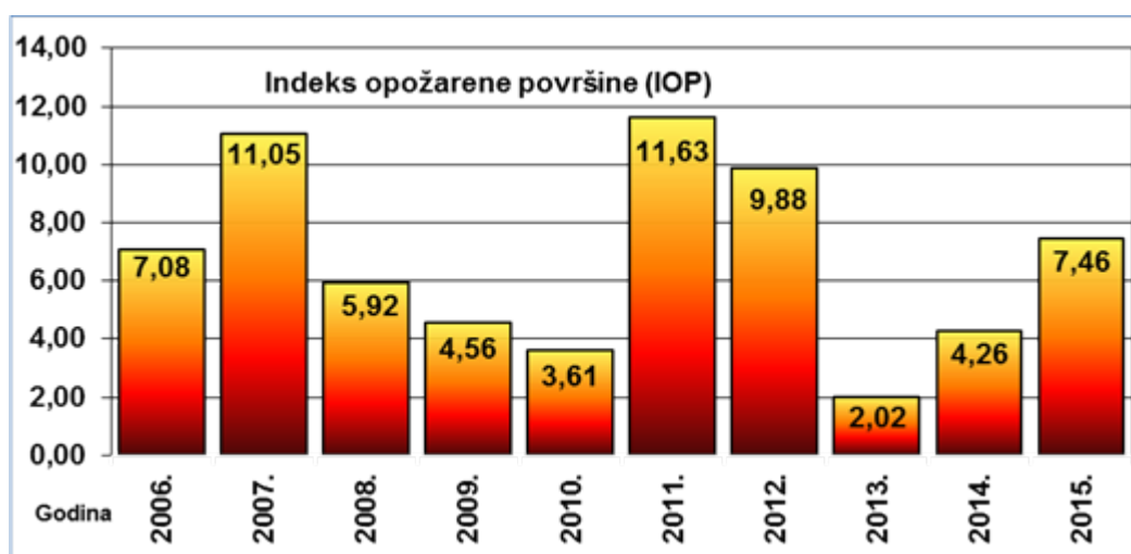
Grafikon 4: IOP za razdoblje 2006. - 2015.
