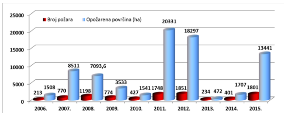
Grafikon 3: broj požara i pripadajuća opožarena površina za razdoblje 2006. – 2015.
